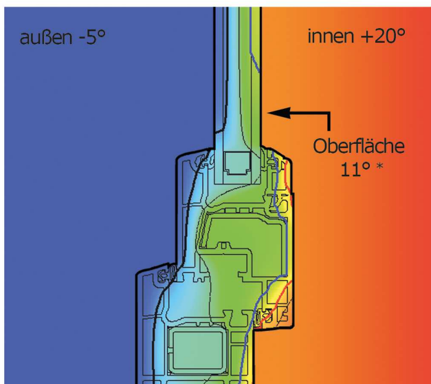
Herkömmliches Fenster
